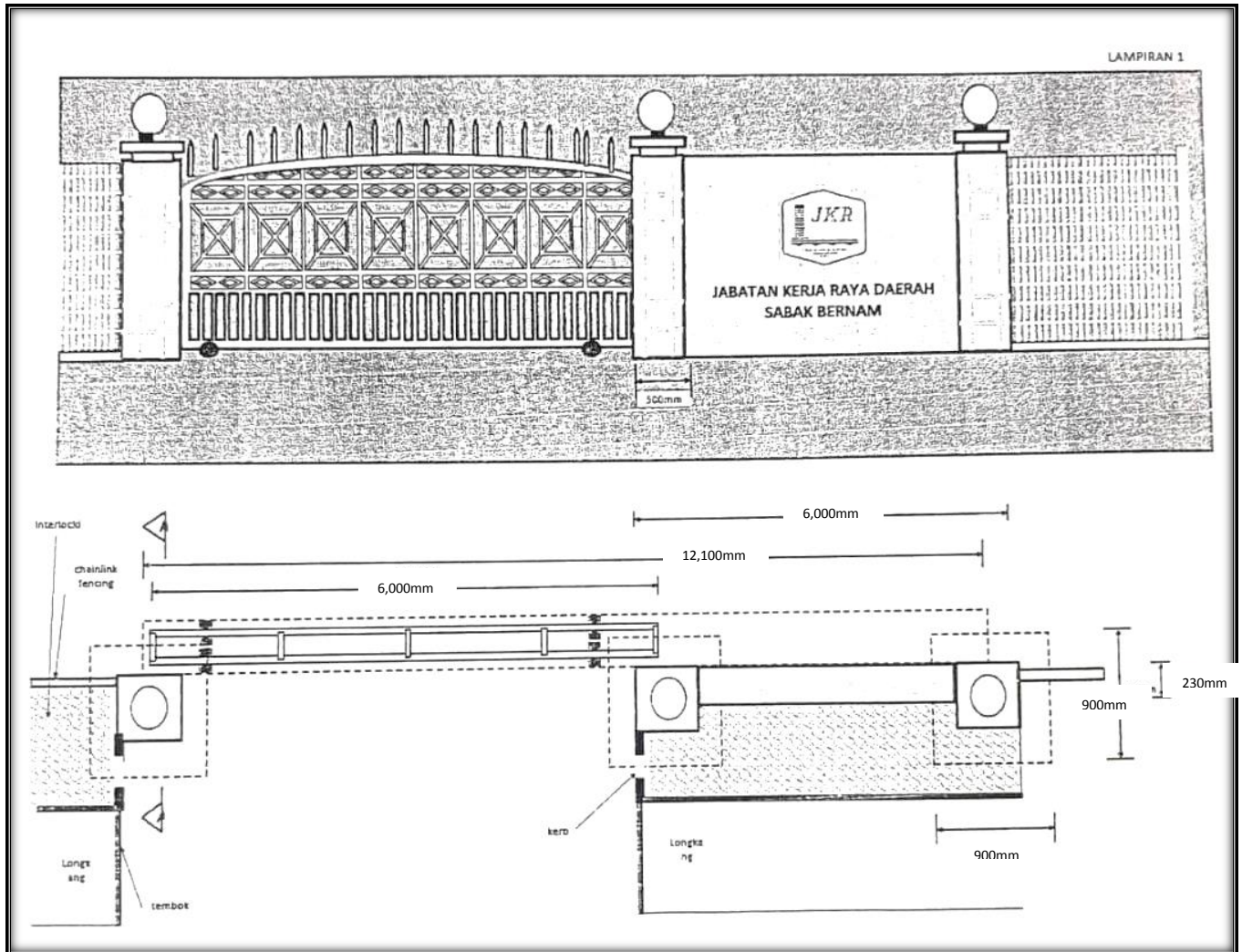
Pintu Pagar Utama Jenis "sliding gate" – LAMPIRAN 1
